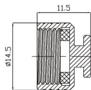
截面A-A Section A-A
