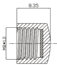
截面 A-A Section A-A
