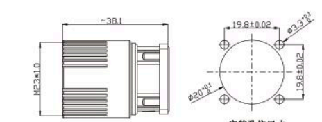
安装孔位尺寸 Mounting dimensions
