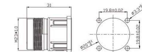
Mounting dimensions 安装孔位尺寸
