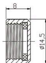
截面 A-A
